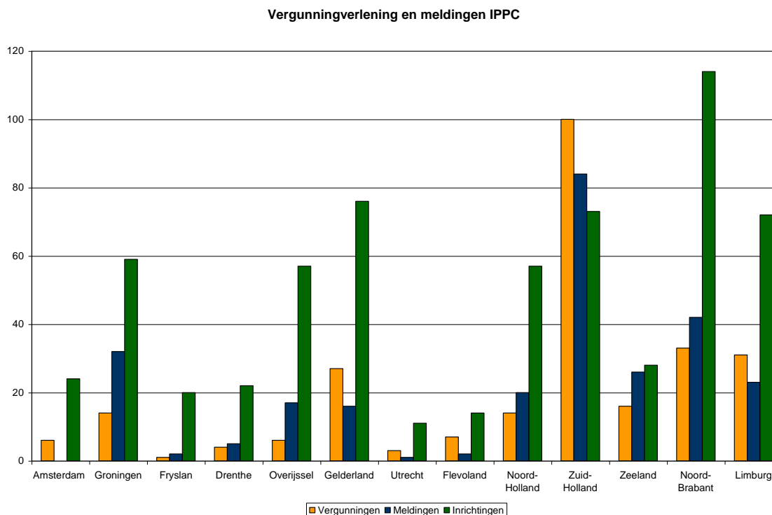
Figuur 13. Vergunningen en meldingen van IPPC bedrijven
